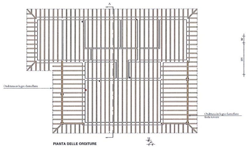
PIANTA DELLE ORDITURE
