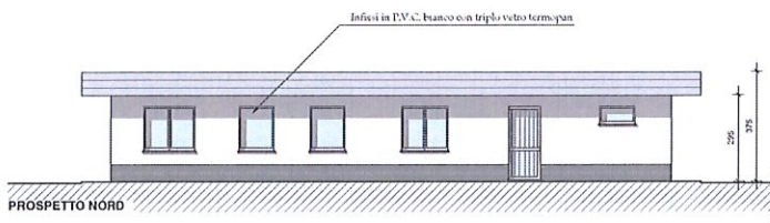
PROSPETTO NORD
