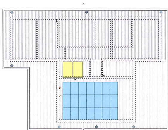
PIANTA DELLA COPERTURA
